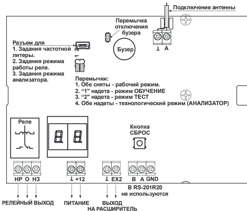
Рис. 6. Монтажная схема приёмника
