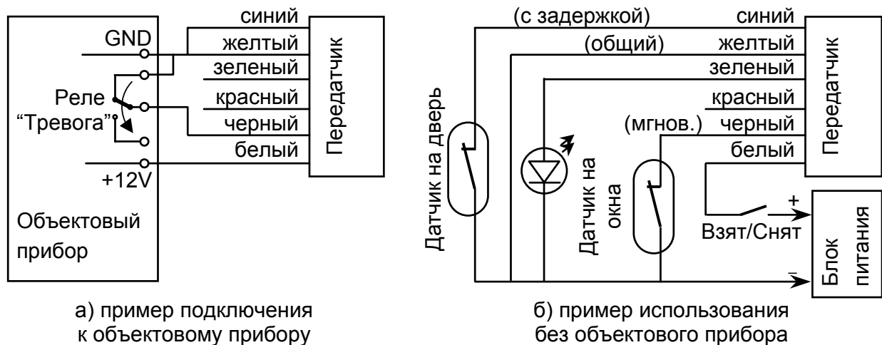
Рисунок 3. Примеры монтажа передатчика
